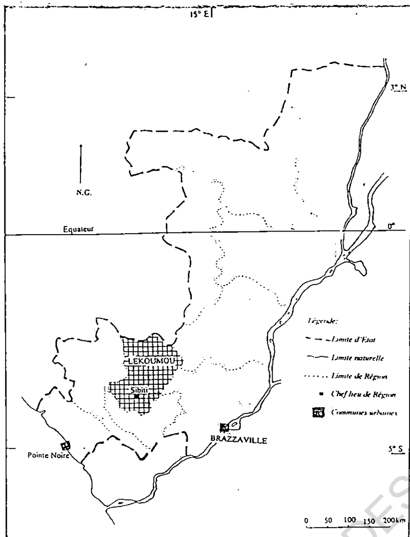
Figure 1: La Lékoumou dans l'espace territorial congolais.
