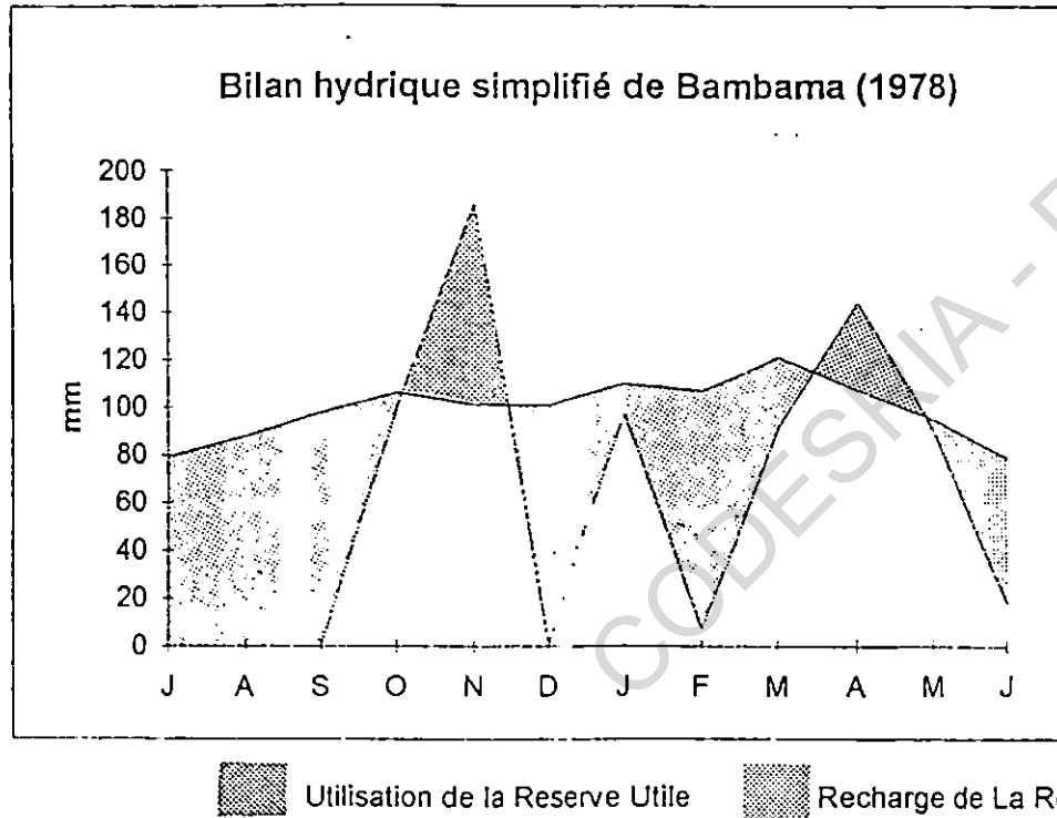
Figure 22 : Bilan hydrique simplifié de quelques années exceptionnelles compté de juillet à juin
